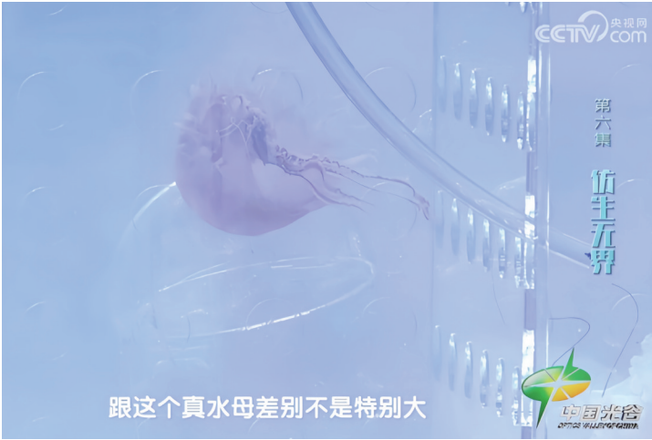
水中遨游的仿生水母机器人。(图片由西北工业大学提供)
